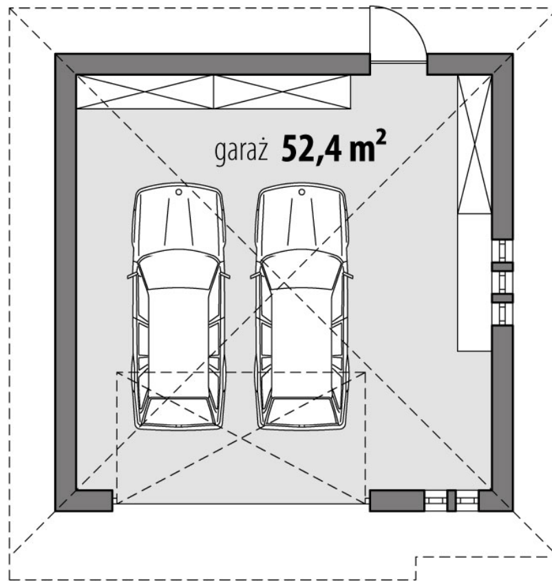
RZUT PARTER
