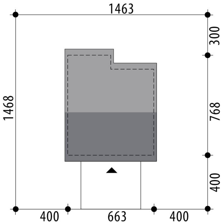
RZUT DZIAŁKI
