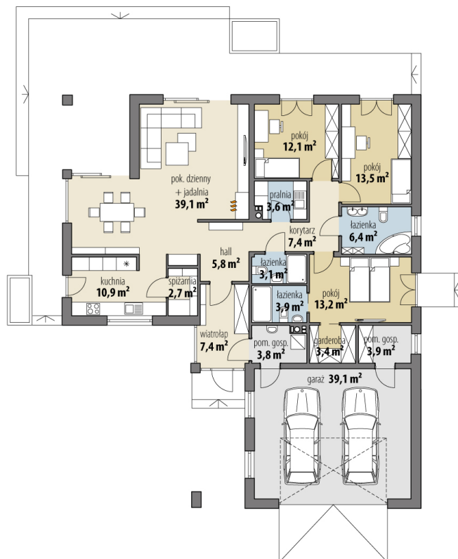
RZUT PARTER
