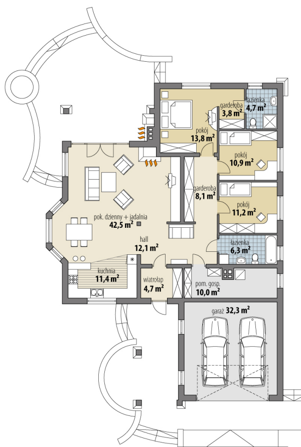
RZUT PARTER
