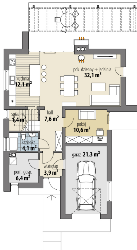
RZUT PARTER
