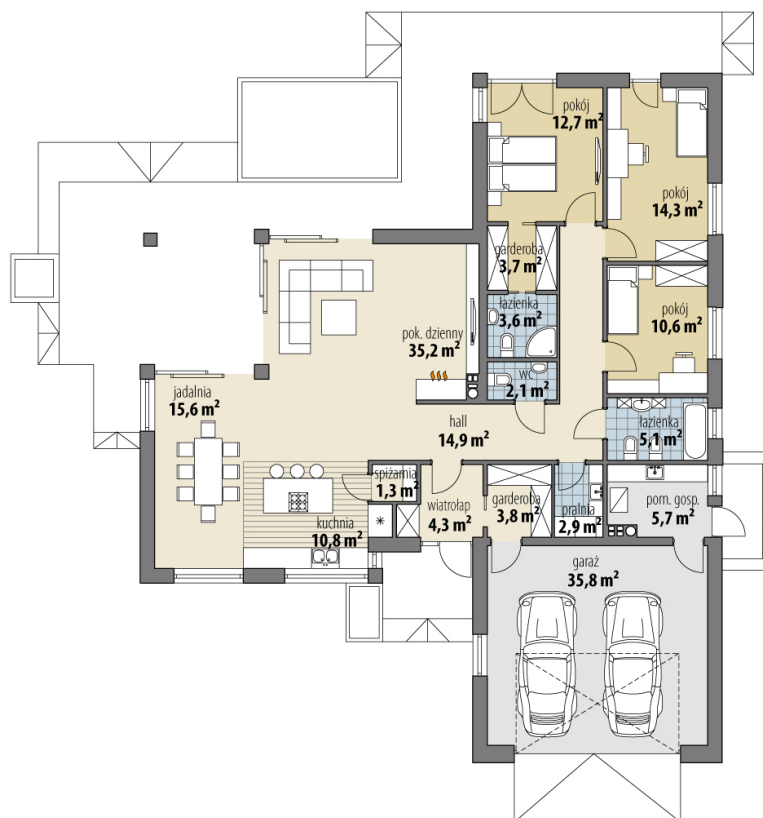
RZUT PARTER
