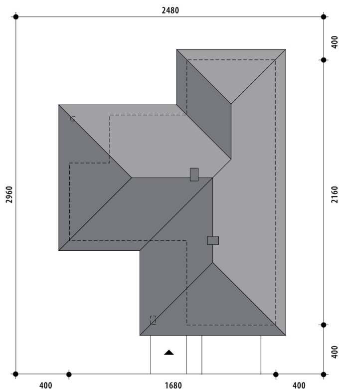
RZUT DZIAŁKI
