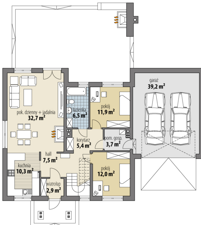
RZUT PARTER
