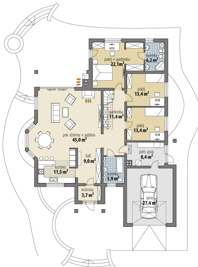
RZUT PARTER
