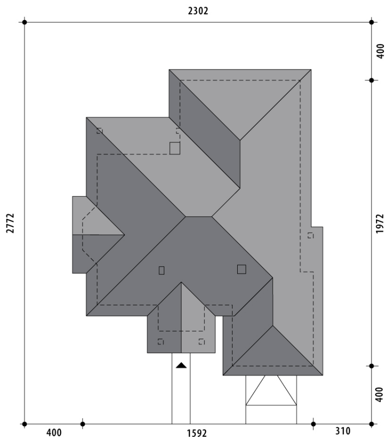
RZUT DZIAŁKI
