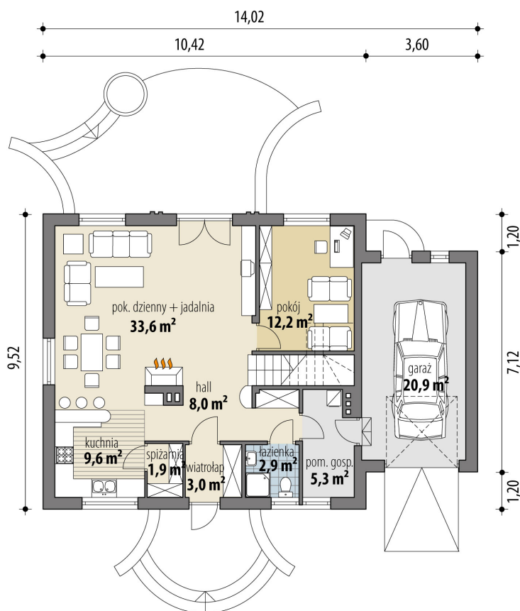
RZUT PARTER
