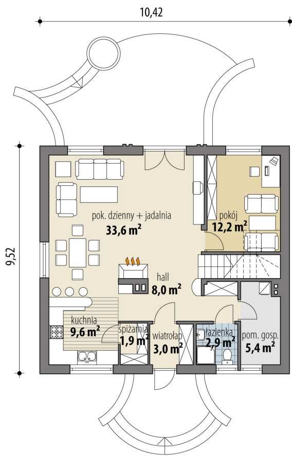
RZUT PARTER
