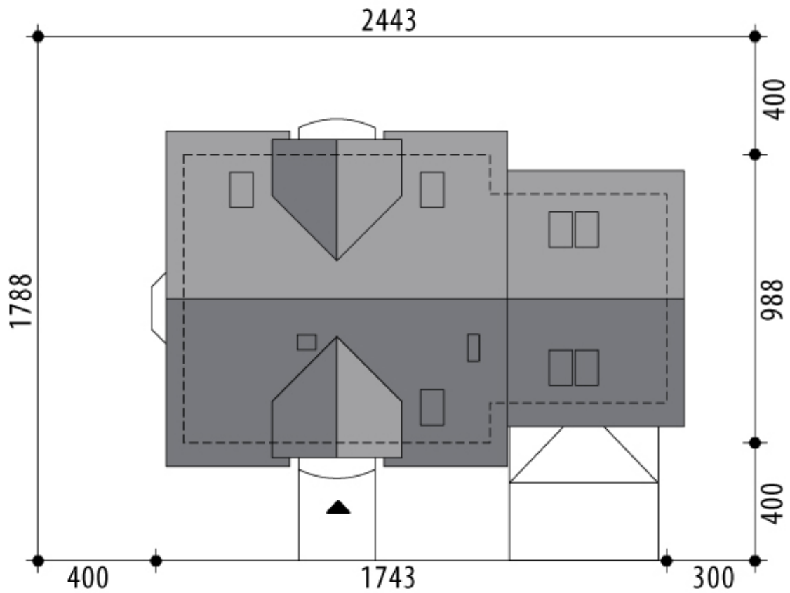
RZUT DZIAŁKI
