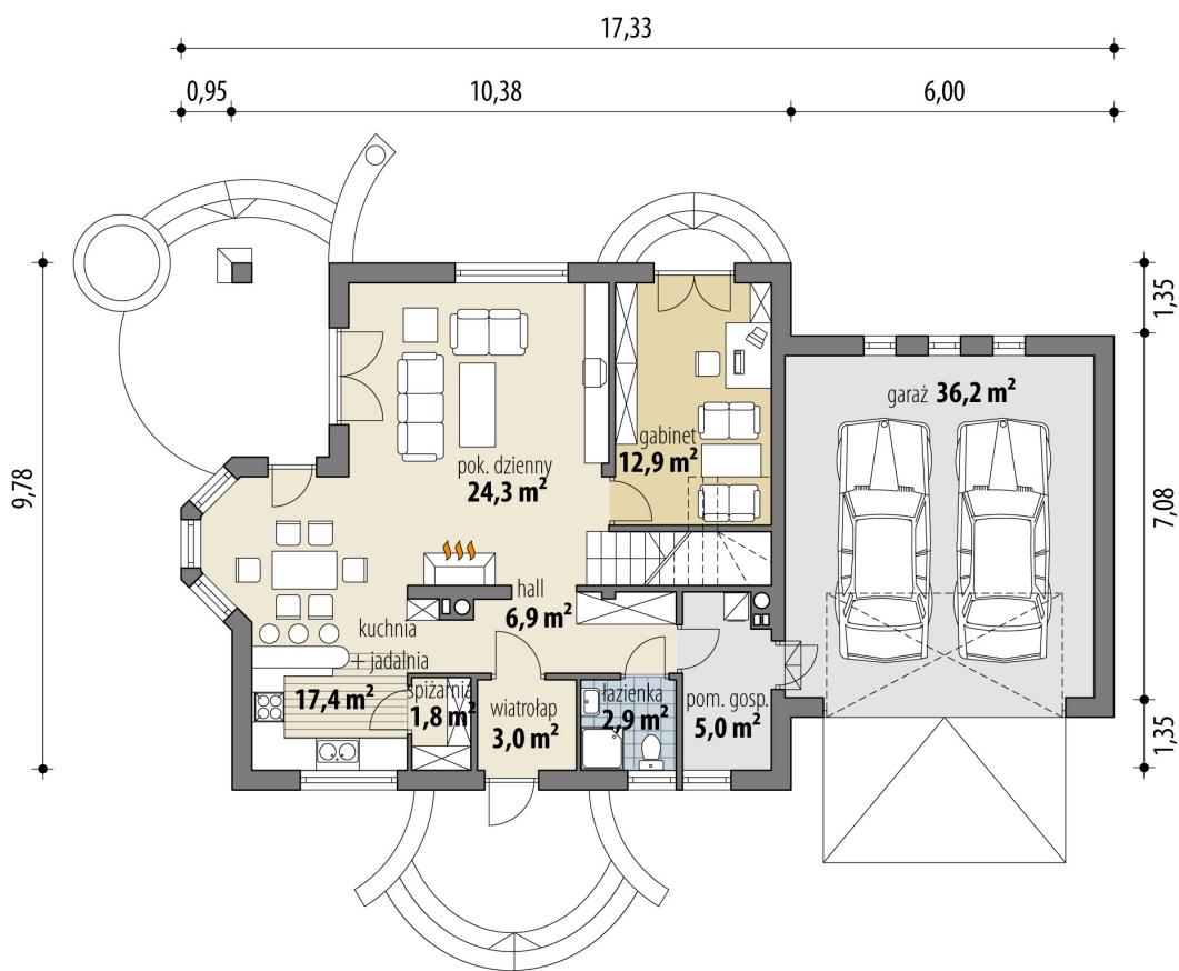
RZUT PARTER
