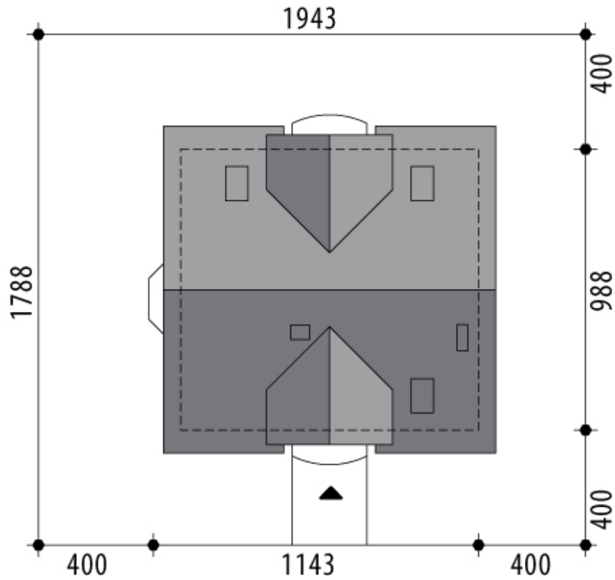
RZUT DZIAŁKI
