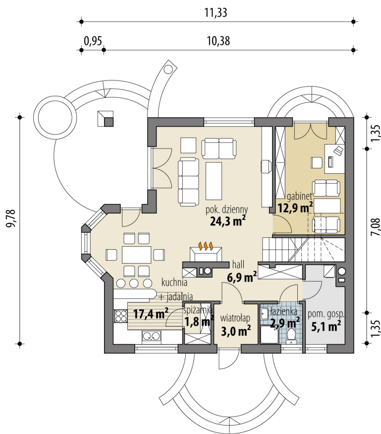
RZUT PARTER
