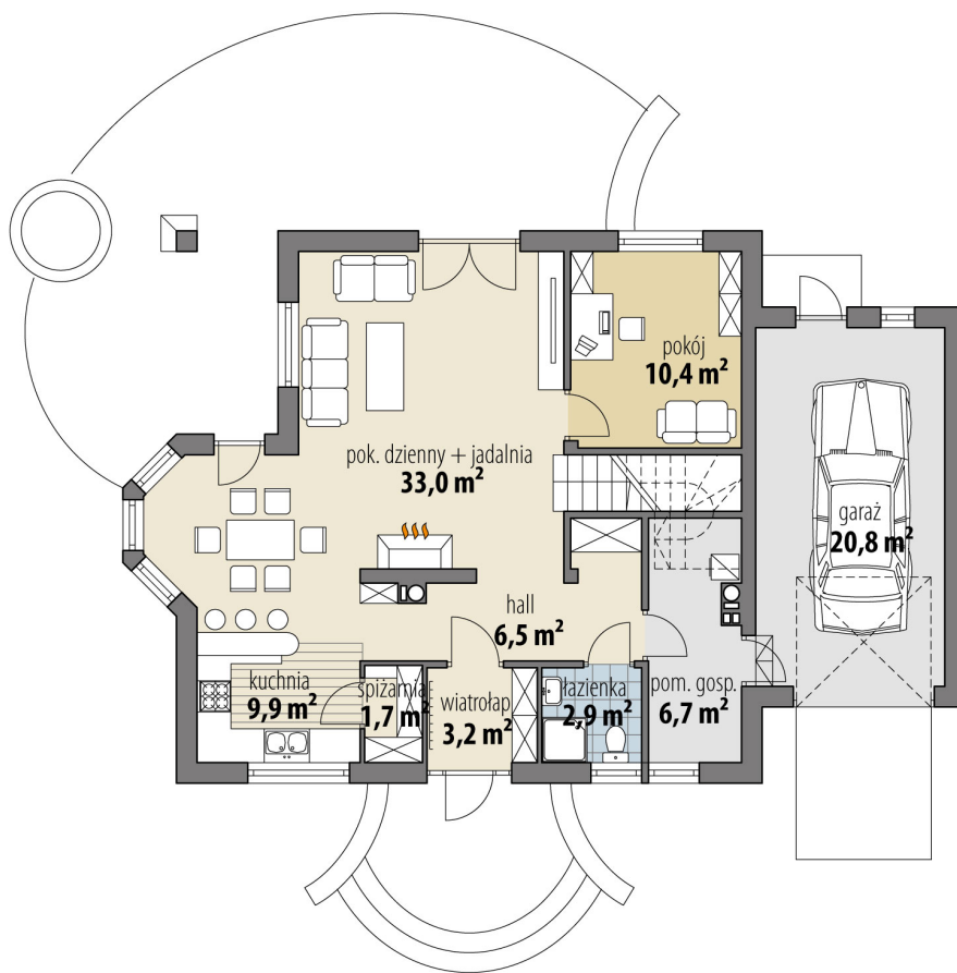
RZUT PARTER
