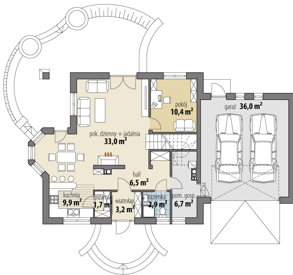
RZUT PARTER
