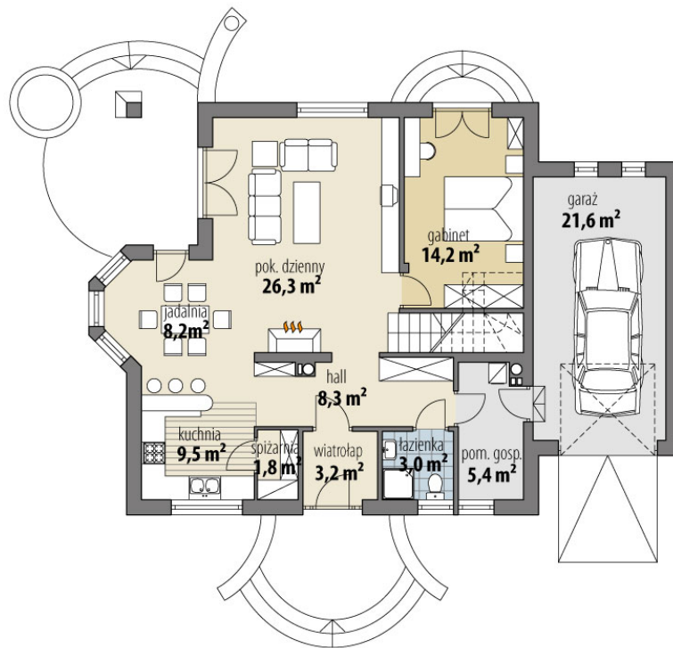
RZUT PARTER
