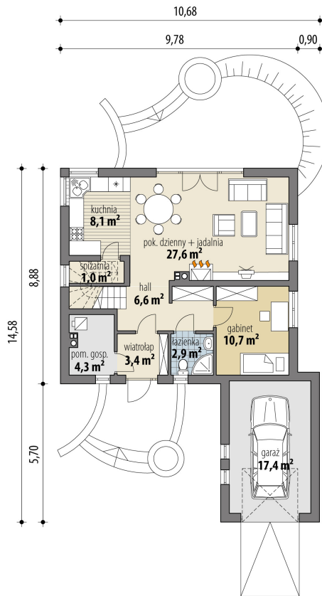
RZUT PARTER
