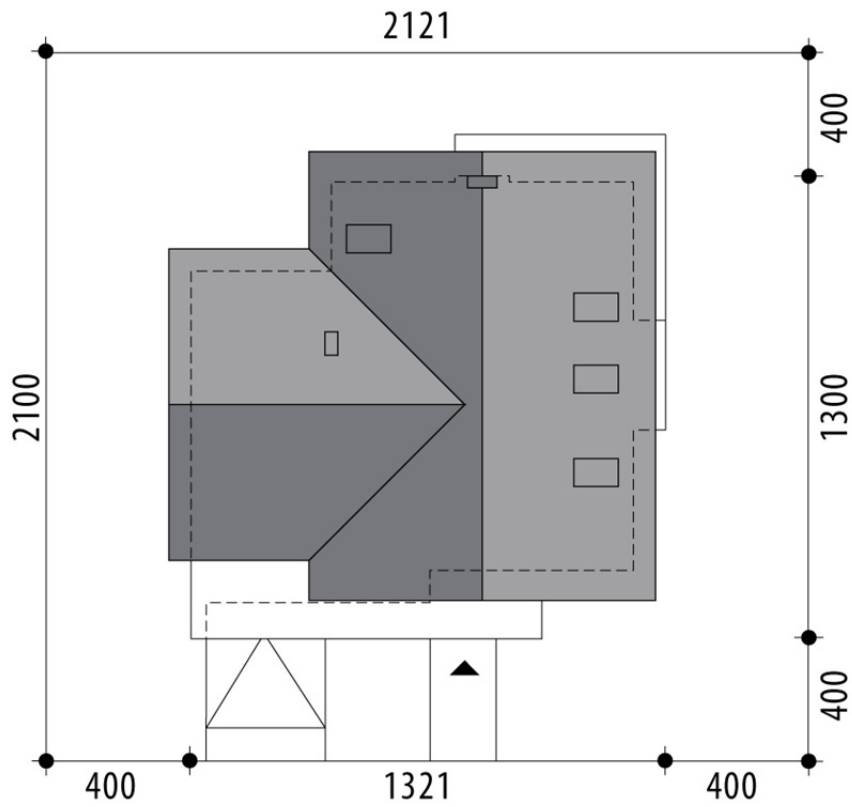
RZUT DZIAŁKI
