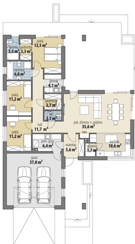
RZUT PARTER
