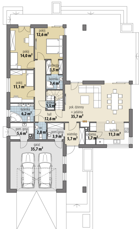
RZUT PARTER
