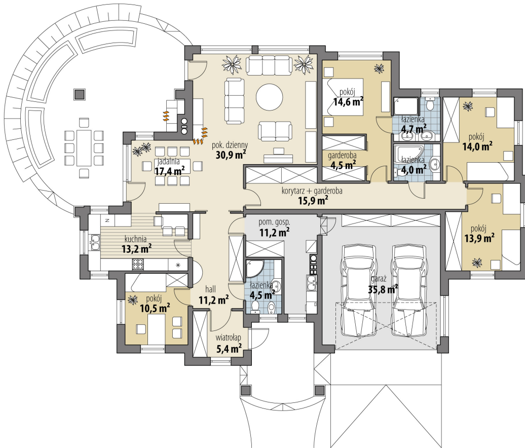
RZUT PARTER
