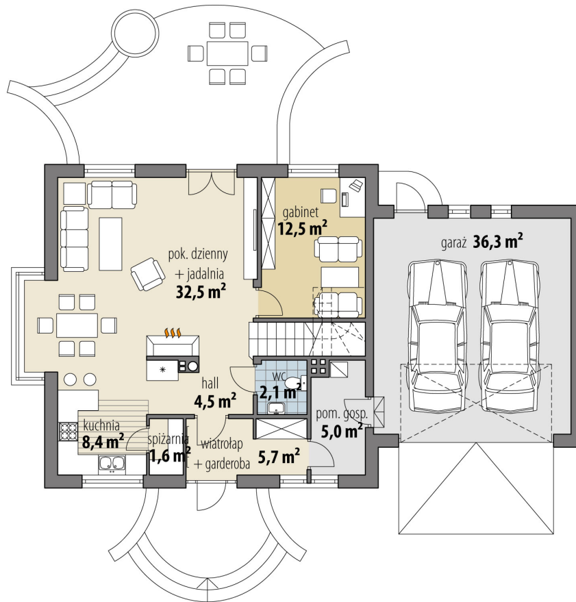
RZUT PARTER
