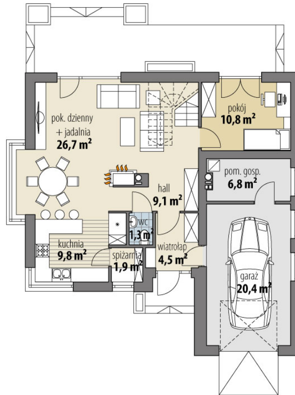
RZUT PARTER
