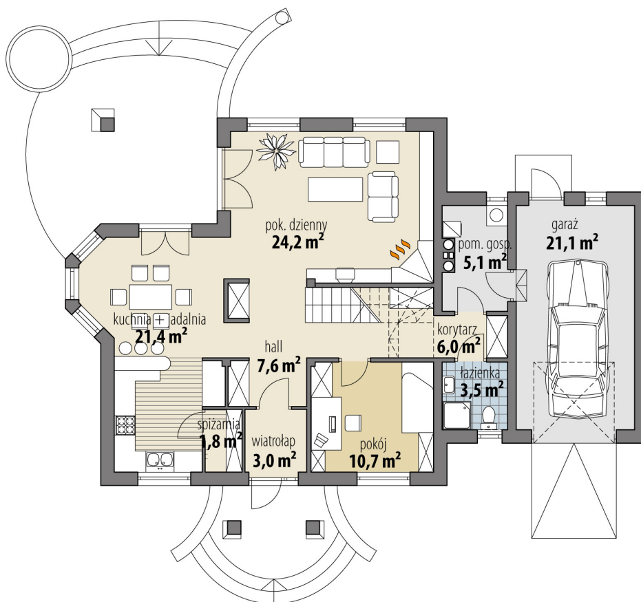
RZUT PARTER
