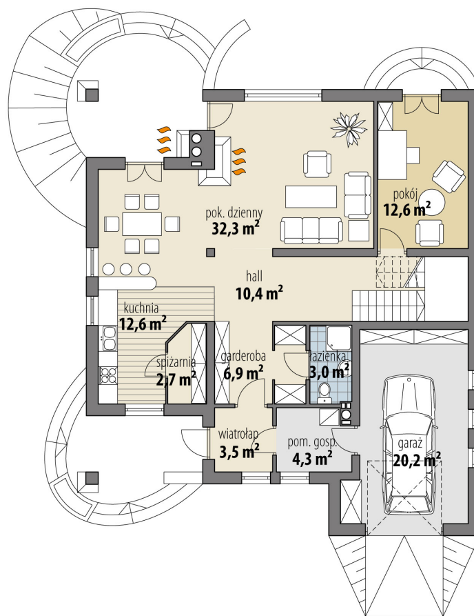
RZUT PARTER
