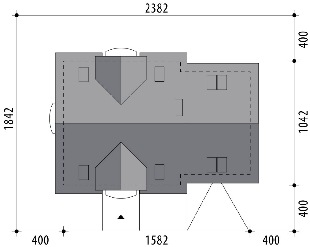
RZUT DZIAŁKI
