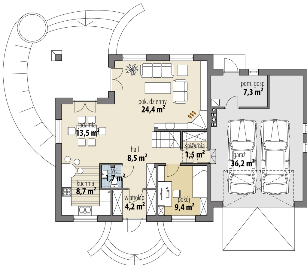
RZUT PARTER
