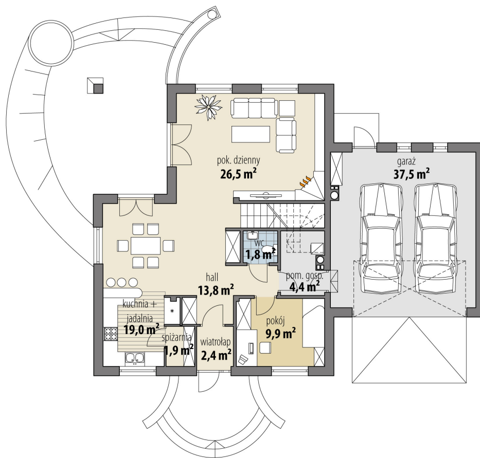
RZUT PARTER
