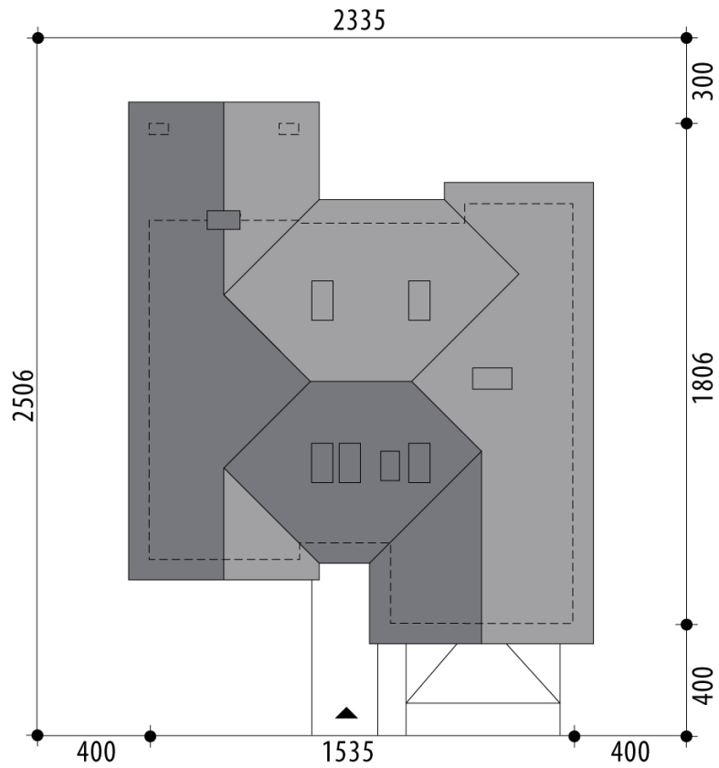
RZUT DZIAŁKI
