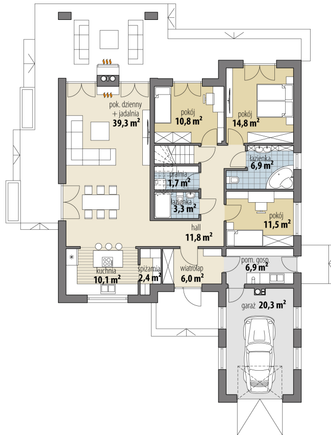
RZUT PARTER
