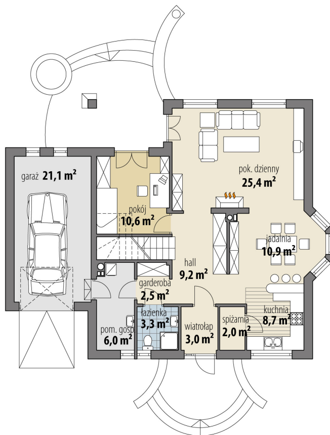
RZUT PARTER
