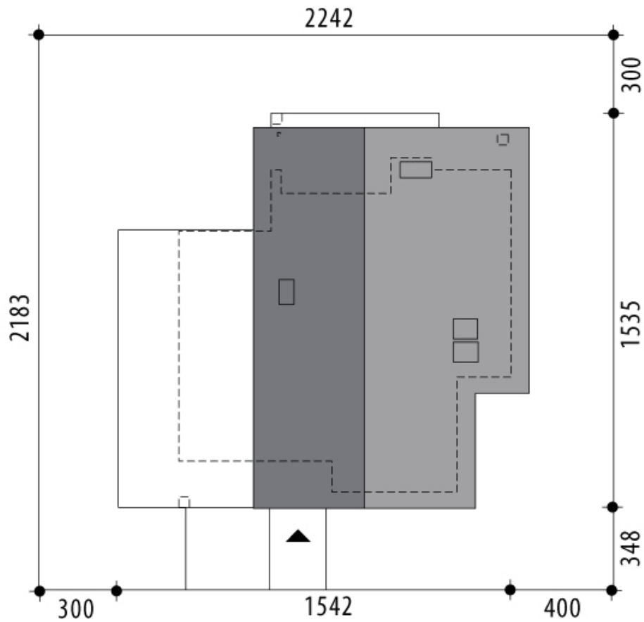
RZUT DZIAŁKI
