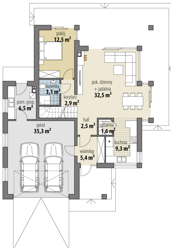
RZUT PARTER
