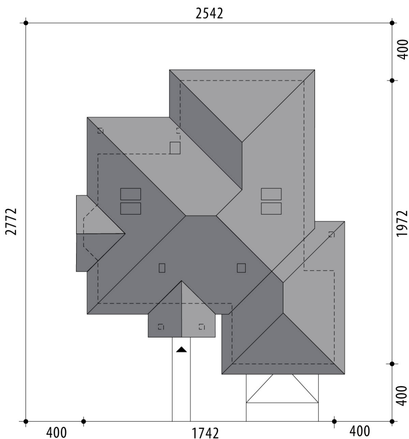
RZUT DZIAŁKI
