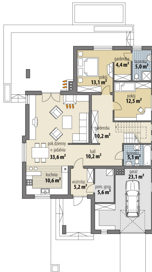
RZUT PARTER
