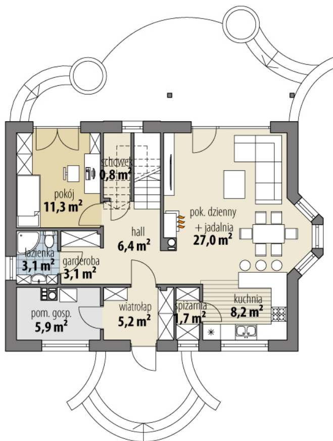
RZUT PARTER
