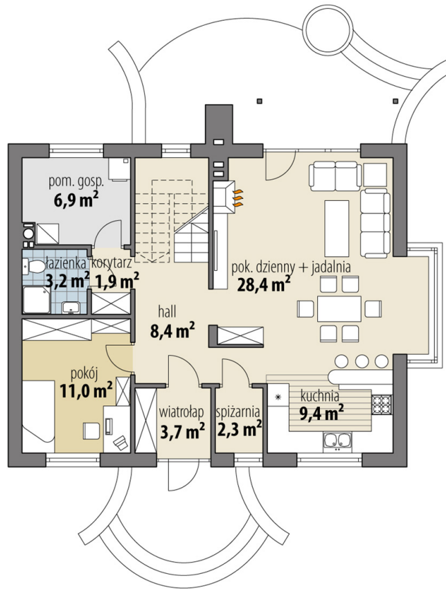
RZUT PARTER
