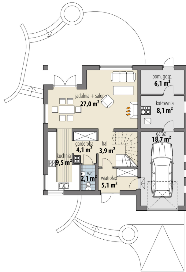
RZUT PARTER
