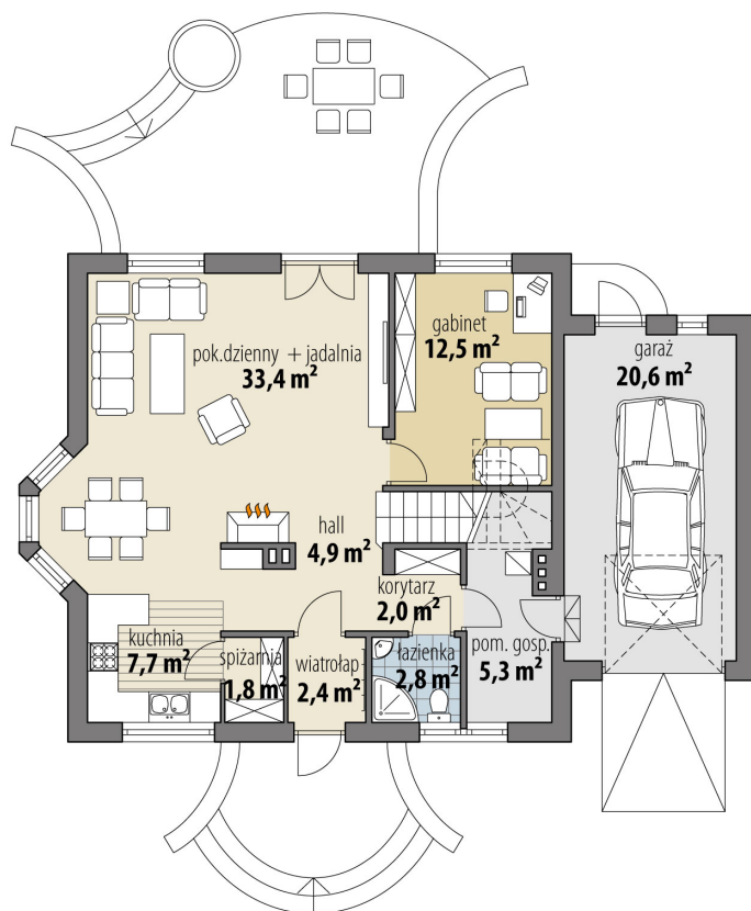
RZUT PARTER
