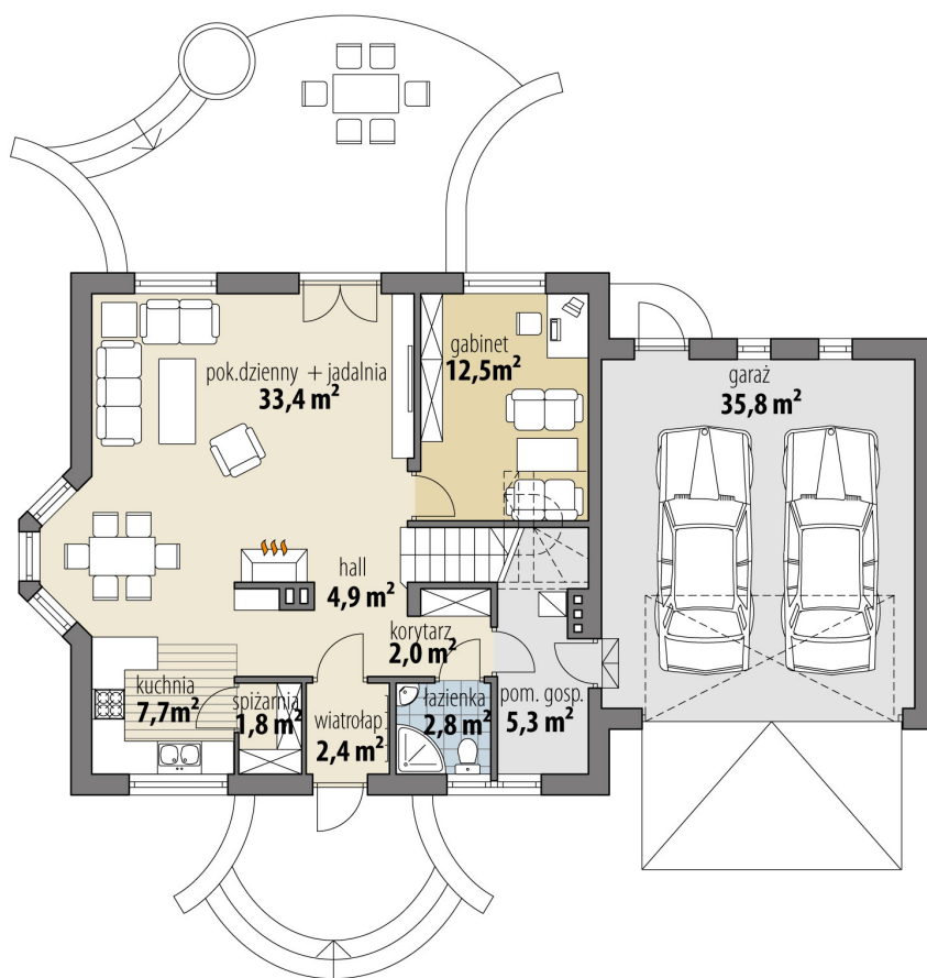
RZUT PARTER
