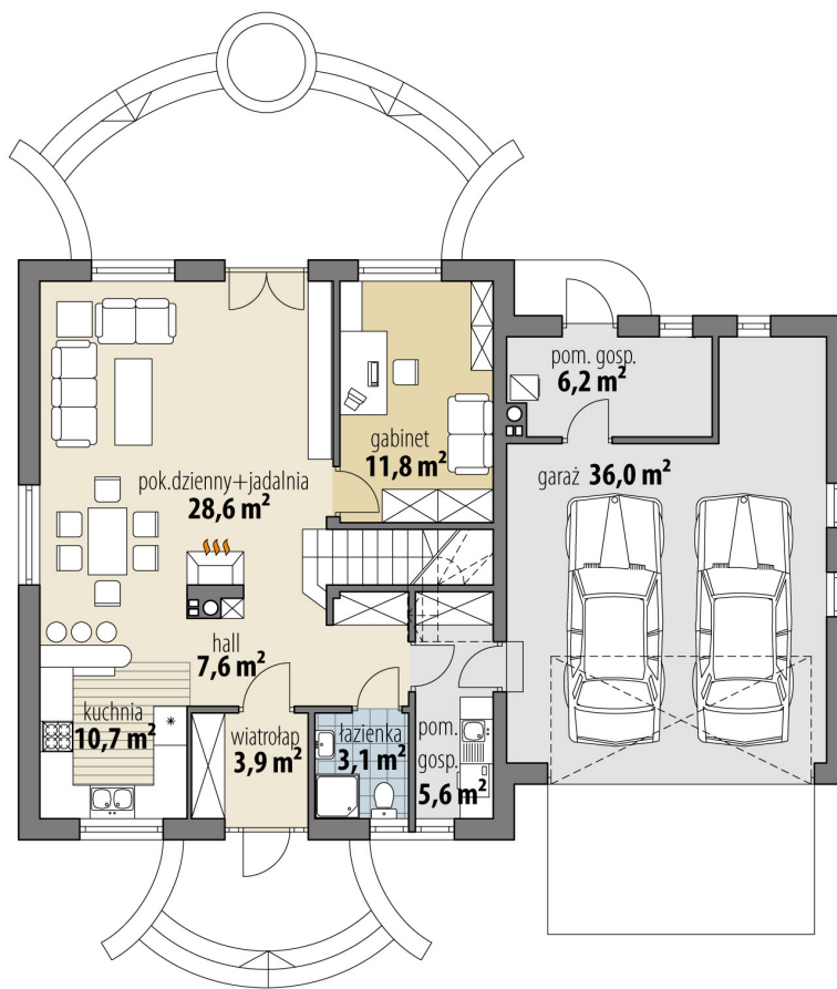
RZUT PARTER
