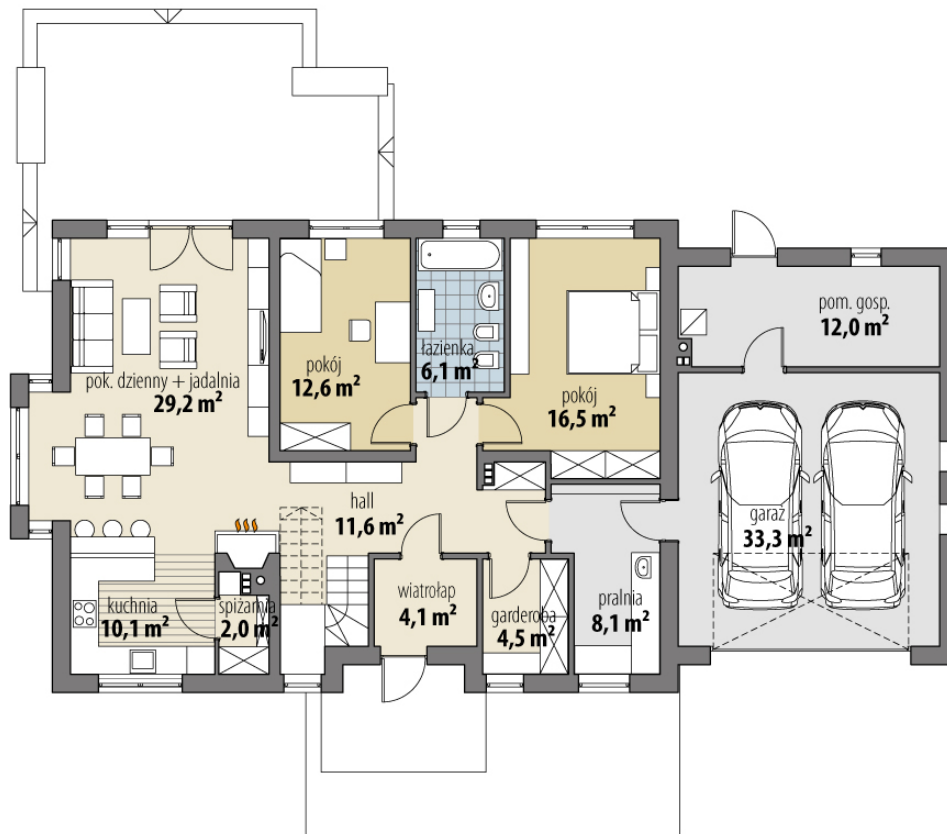
RZUT PARTER
