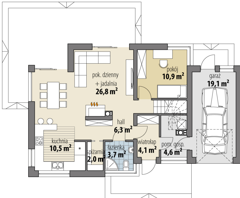
RZUT PARTER
