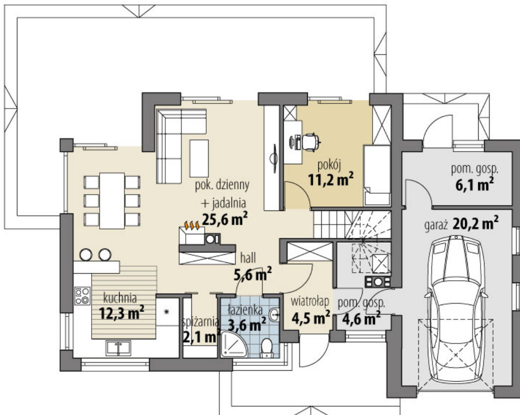
RZUT PARTER
