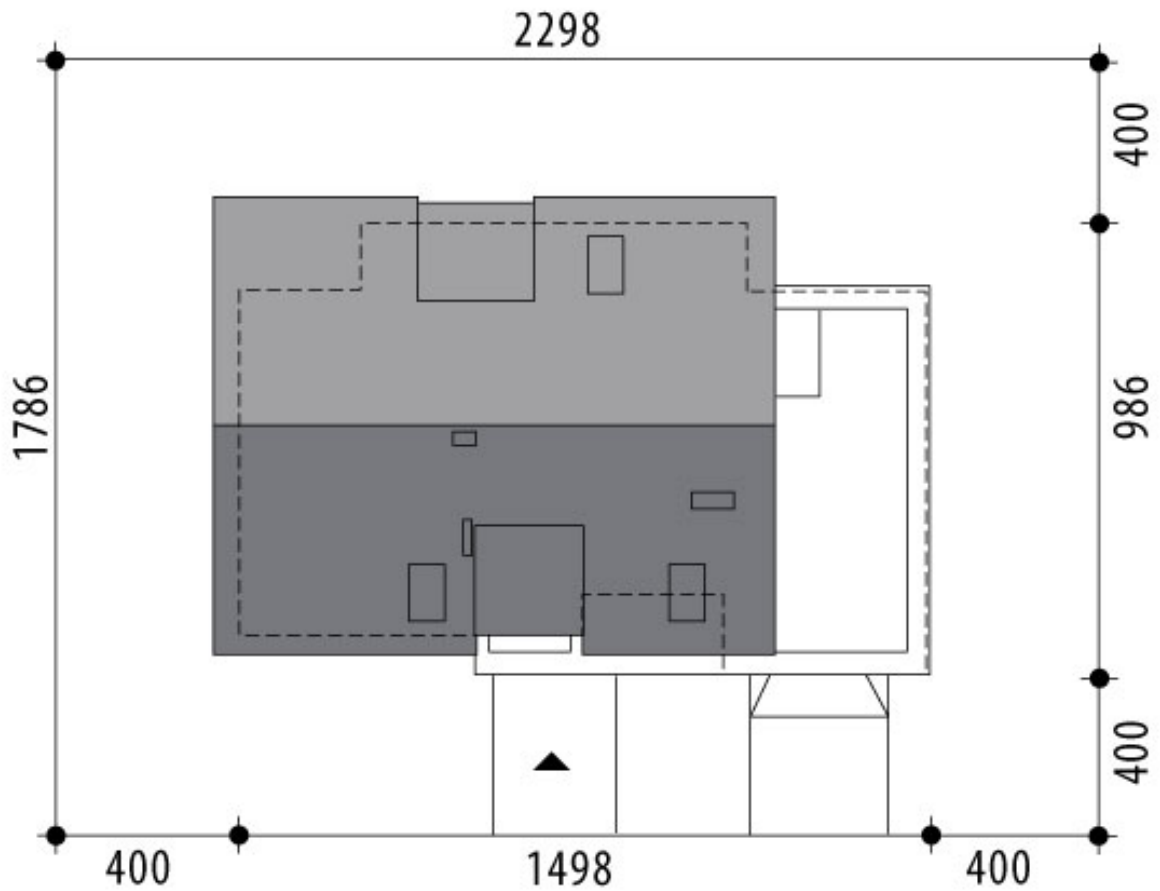
RZUT DZIAŁKI
