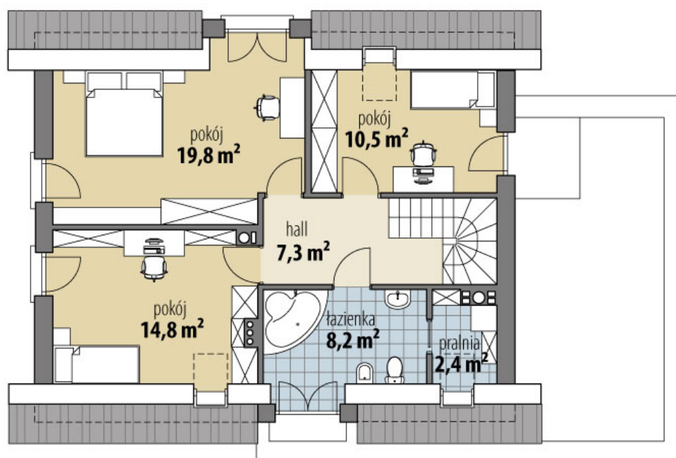
RZUT
