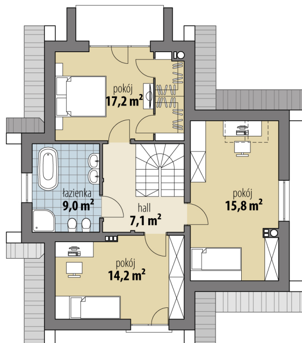
RZUT
