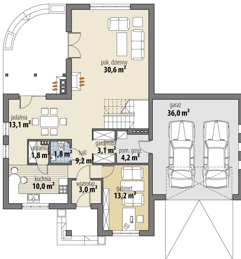
RZUT PARTER
