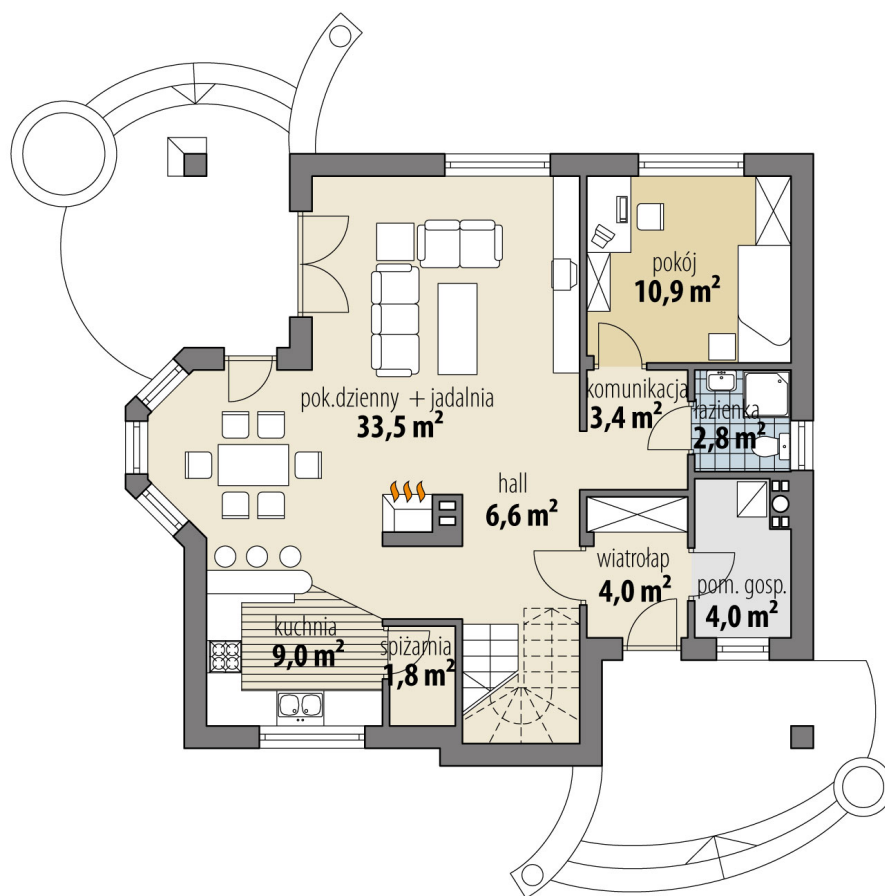
RZUT PARTER
