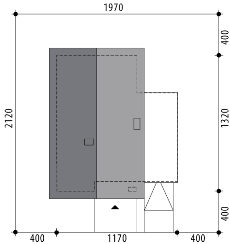
RZUT DZIAŁKI
