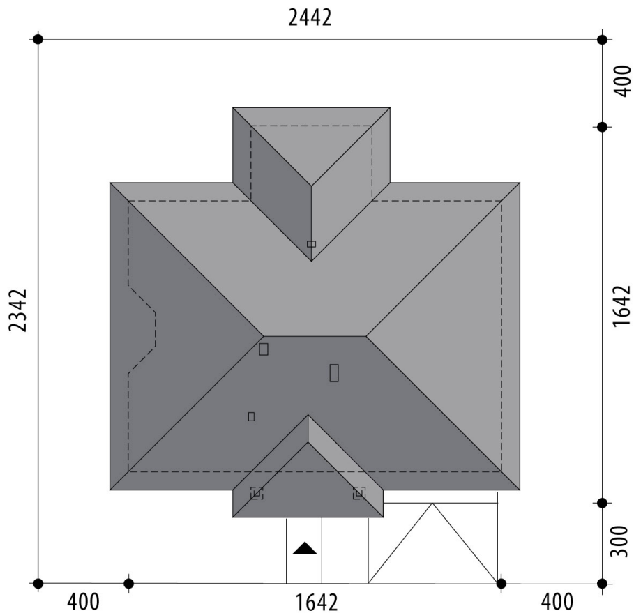
RZUT DZIAŁKI
