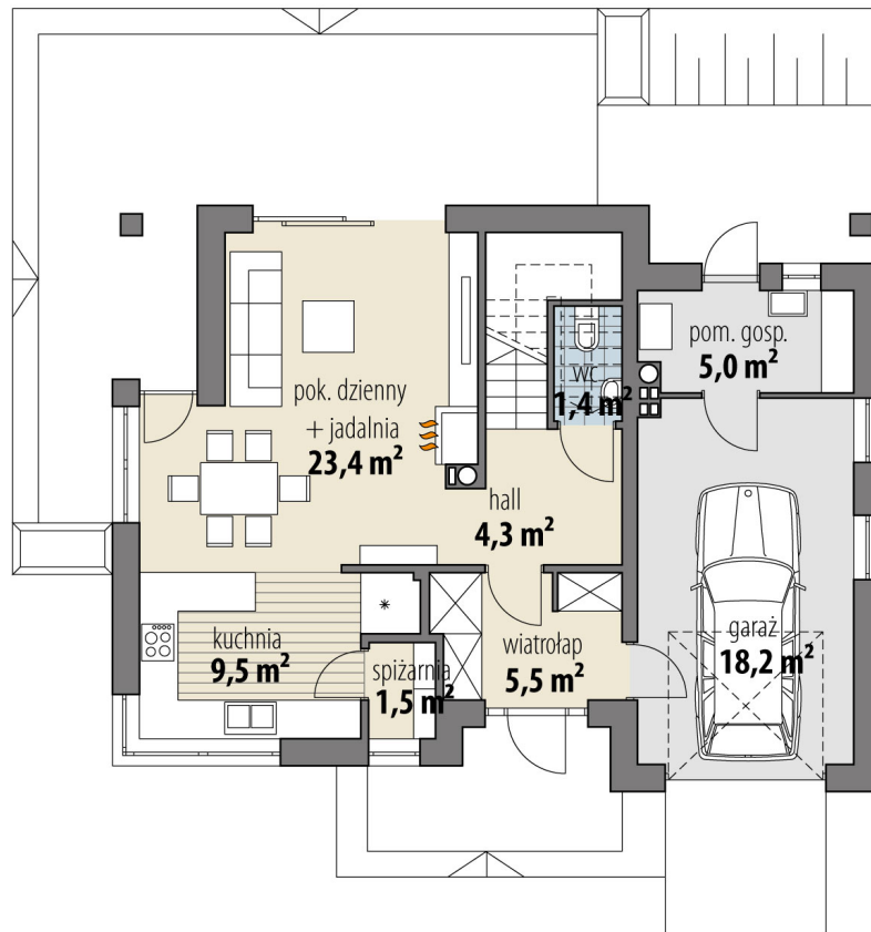
RZUT PARTER
