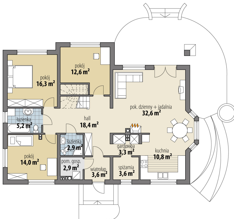
RZUT PARTER
